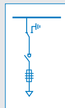
Выключатель нагрузки с предохранителем
