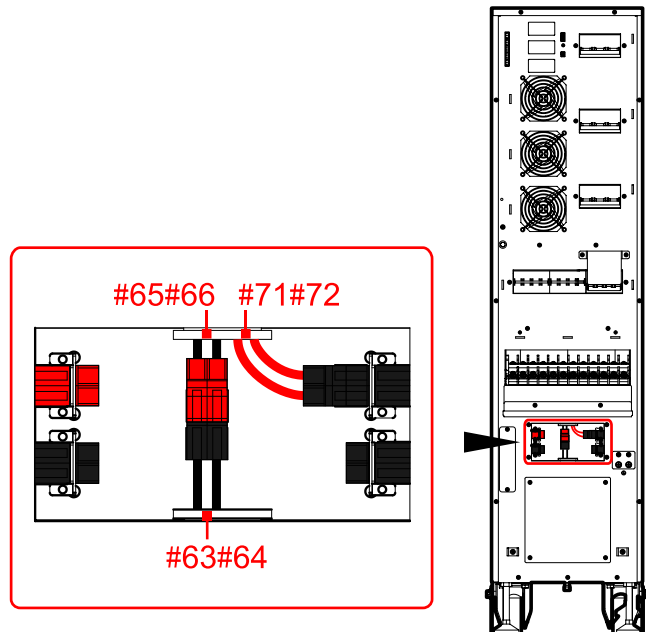
Рис. 3-20 Режим клемм коннектора по умолчанию
