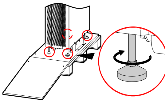
Рис. 3-5 Опорные ножки
