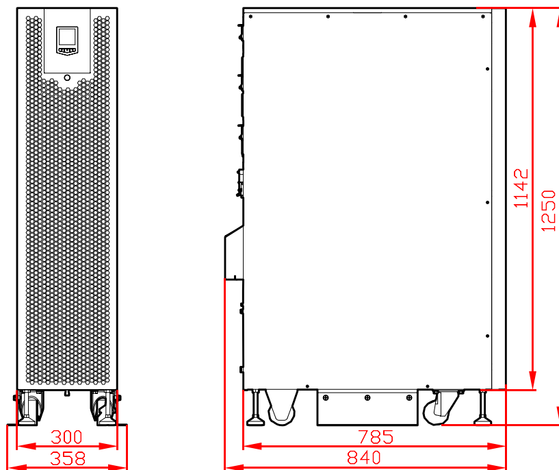
Рис. 3-7 Внешние размеры ИБП VGD-II-30K33HC / VGD-II-30K33HCS / VGD-II-30K33HCT / VGD-II-40K33HC / VGD-II-40K33HCS / VGD-II-40K33HCT (единица измерения: мм)
