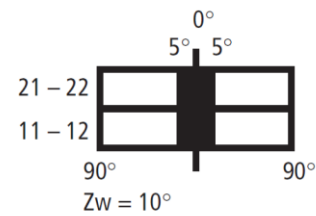
Диаграмма переключения
