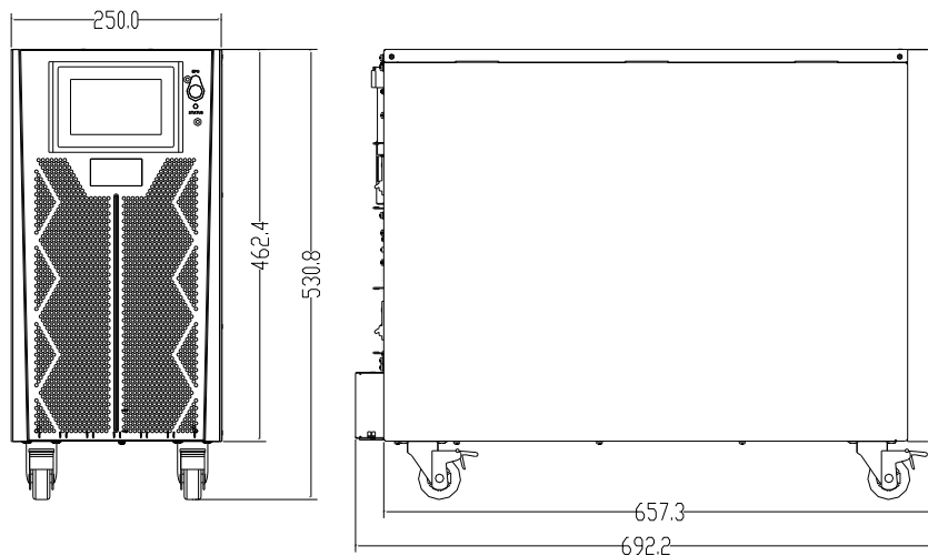
Рисунок 8 (а) Размеры ИБП 10-15 КВА (мм)
