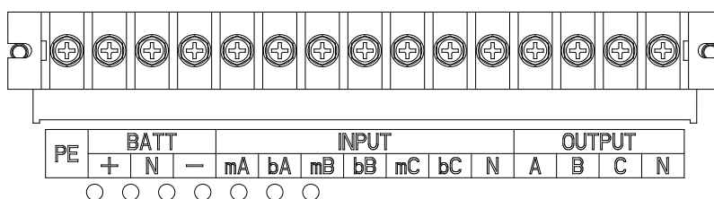
Рисунок 15. Терминалы для подключения кабелей моделей 10/15kVA
