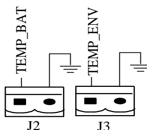
Рисунок 19. Контакты J2 и J3 для определения температуры
