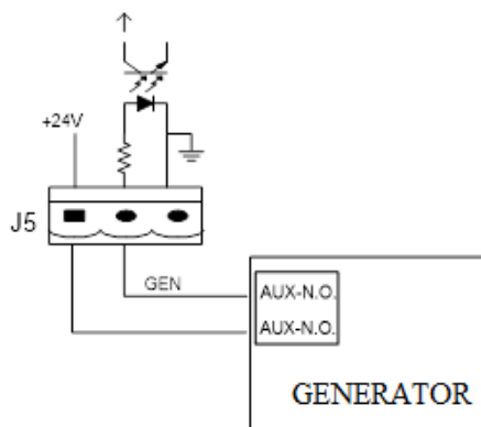
Рисунок 21. Контакт питание ИБП осуществляется от генератора
