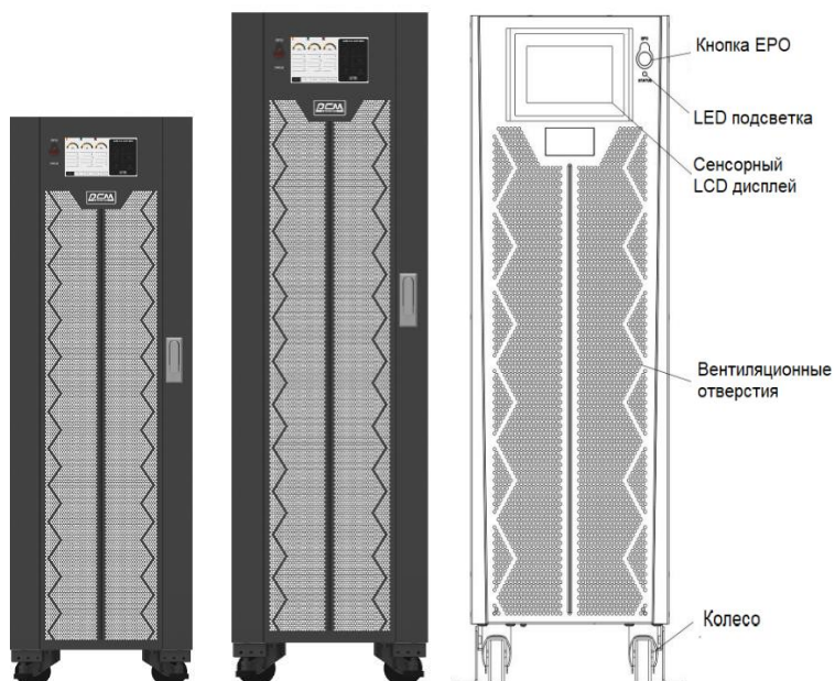
Рисунок 1. (а) Внешний вид ИБП 10-40 КВА (вид спереди)
