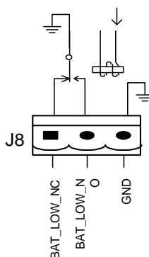
Рисунок 23. Сухой контакт сигнала о низком заряде АКБ
