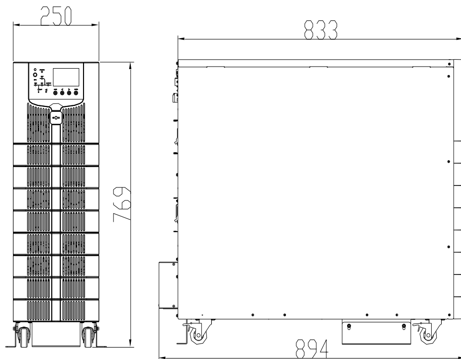
Рисунок 8 (в) Размеры ИБП 40 КВА (мм)
