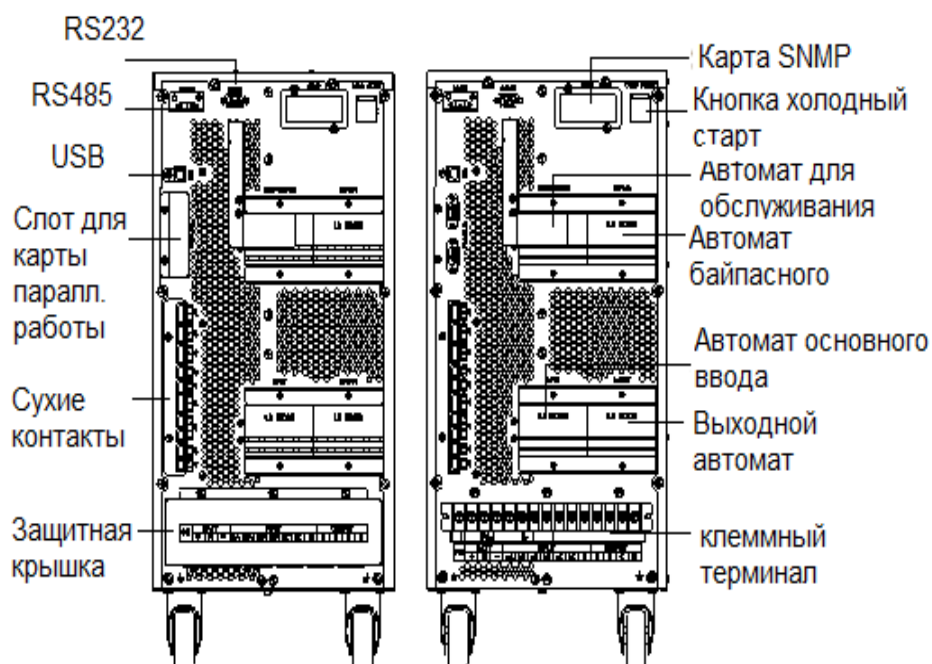
Рисунок 1. (б) Внешний вид ИБП 10-15 КВА (вид сзади)
