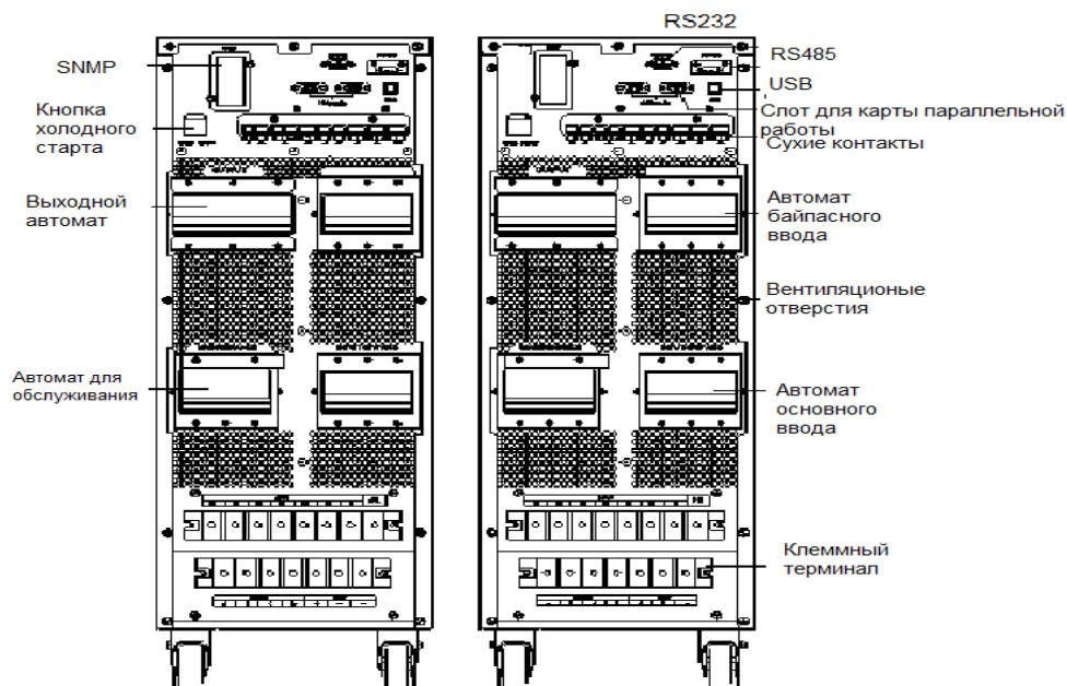
Рисунок 1. (в) Внешний вид ИБП 20-30 КВА (вид сзади)
