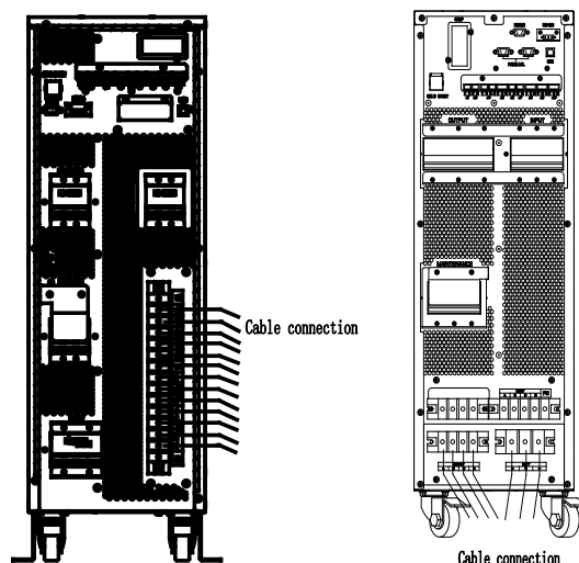
Рисунок 14. Кабельные вводы
