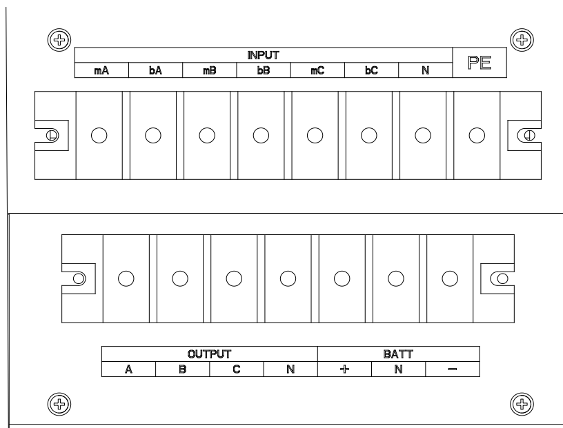
Рисунок 17. Терминалы для подключения кабелей моделей 40kVA
