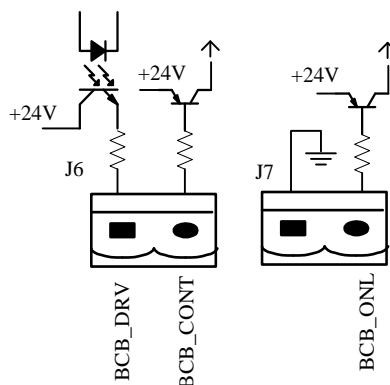
Рисунок 22. Контроль VCB (управление автоматическим выключателем АКБ)
