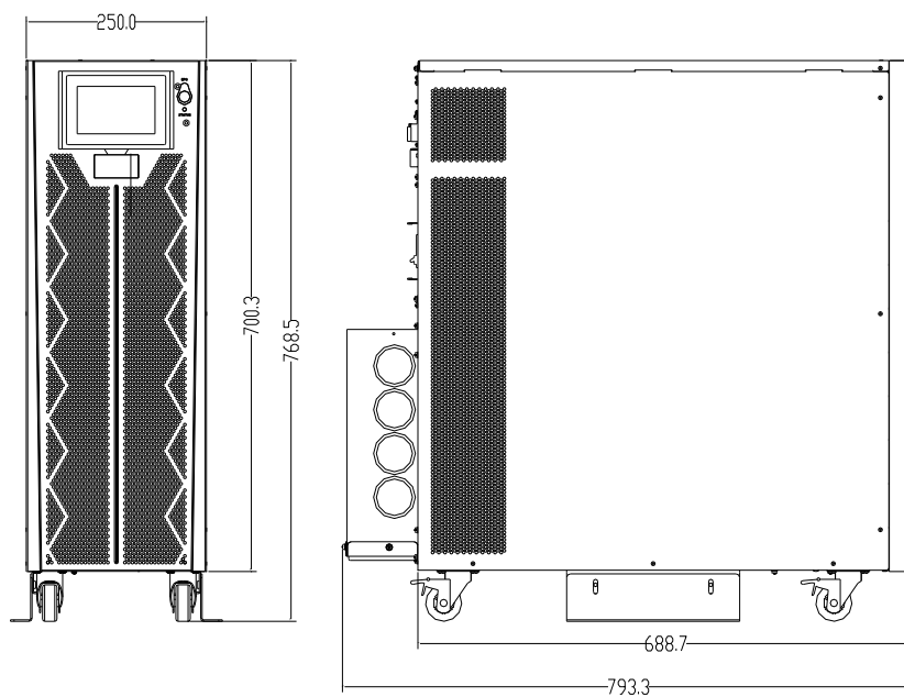
Рисунок 8 (б) Размеры ИБП 20-30 КВА (мм)
