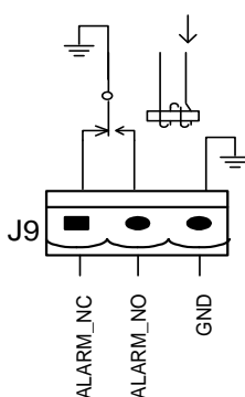
Рисунок 24. Сигнализация об аварии (общий)
