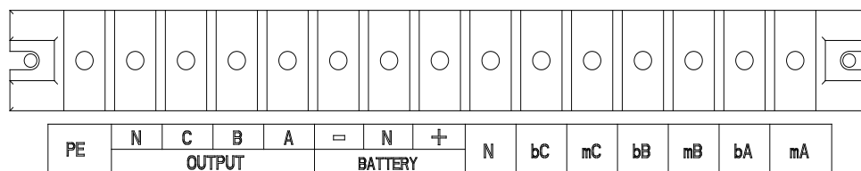
Рисунок 16. Терминалы для подключения кабелей моделей 20/30kVA
